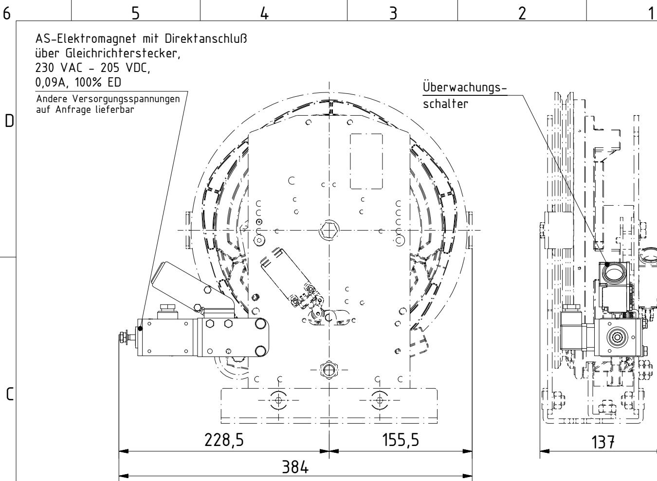
Anbaubeispiel: HJ 300 SB U
